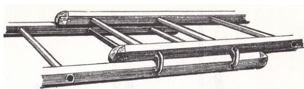
Skarv av stålstegar och trästegar
