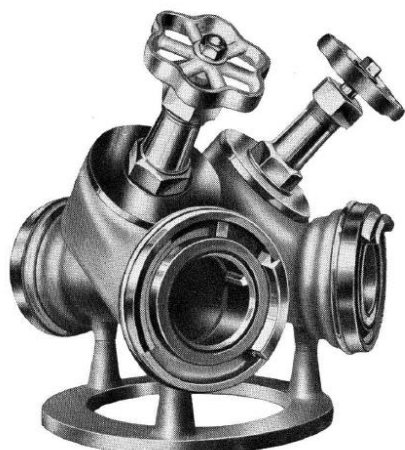
N:r 205. Grenrör med 63×63×63 mm. normalkopplingsanslutning. Ventilavstängning och ringföt.
